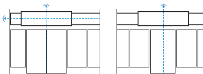
schematy umieszczania kasetonów i paneli poziomych na fryzie budynku
